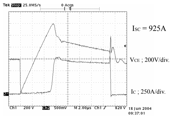
Fig. 6 V GE =18V
